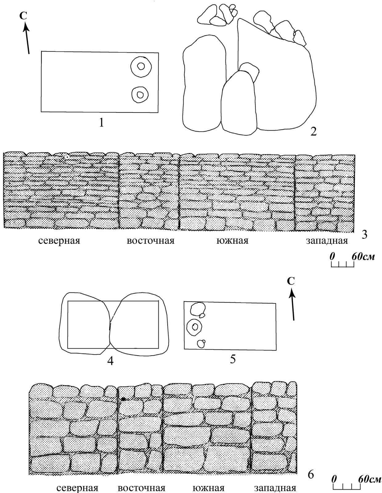
Рис 31. Подкурганые склепы могильника Гентал у с.Кафыркумух. Планы и профили стенок склепов №1 и №2. По М.Г. Магомедову
