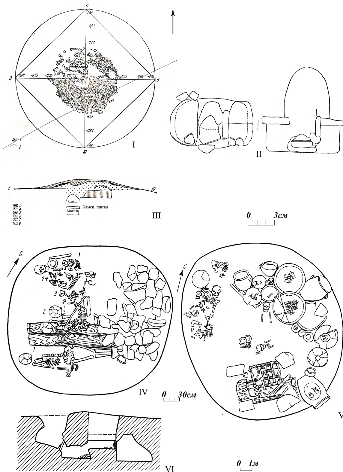
Рис 30. Подкурганые могилы и катакомбы у ст. Манас. I – план кургана 1; II – план разрез могилы со сводом; III – профиль кургана по линии С–Ю; IV–VI – планы и профили захоронений в катакомбах 1 и 2 кургана 3. По К.Ф. Смирнову и Р.М. Мунчаеву
