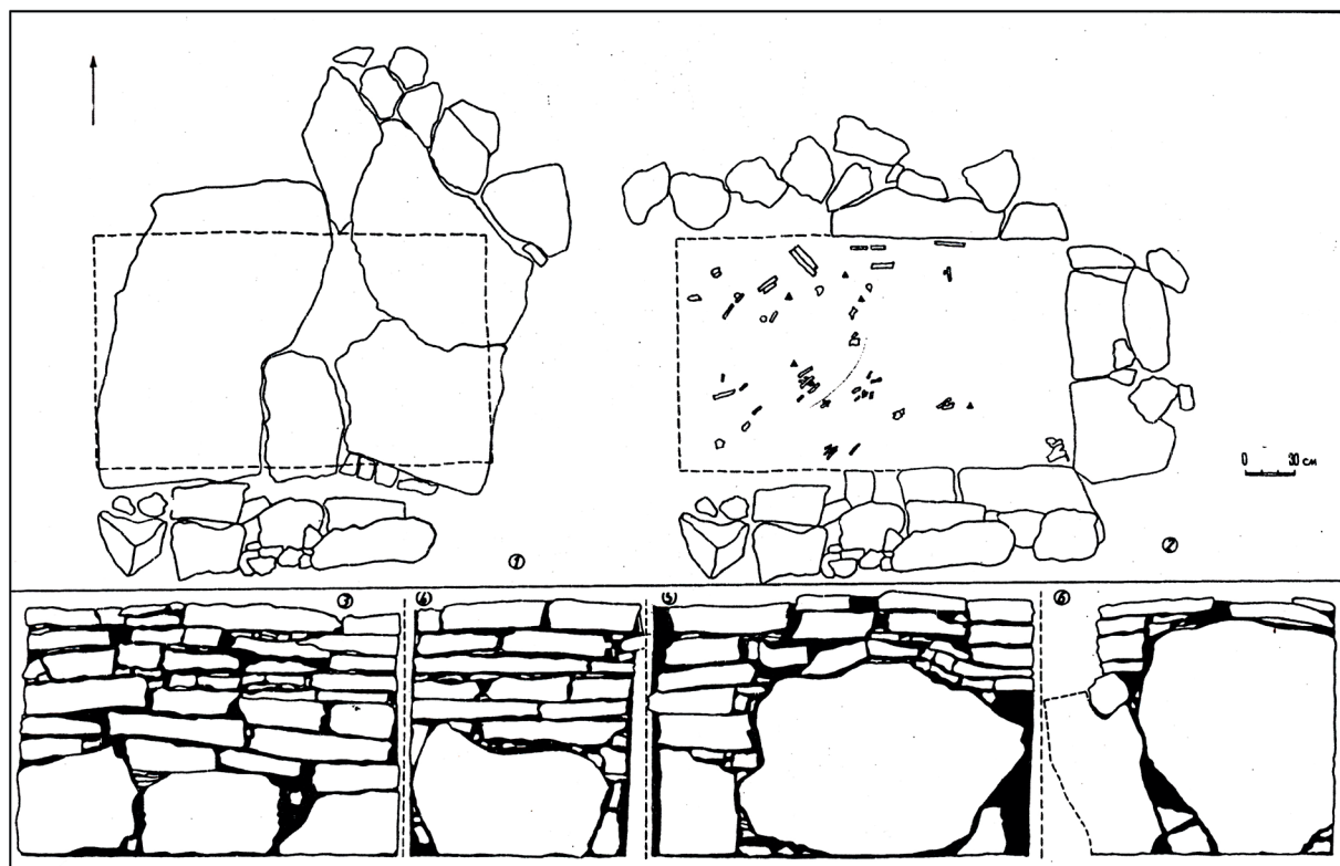
Рис 20. Могильник Муги. Склеп №1: планы (1–2) и профили стен (3–6). По Р.М. Мунчаеву
