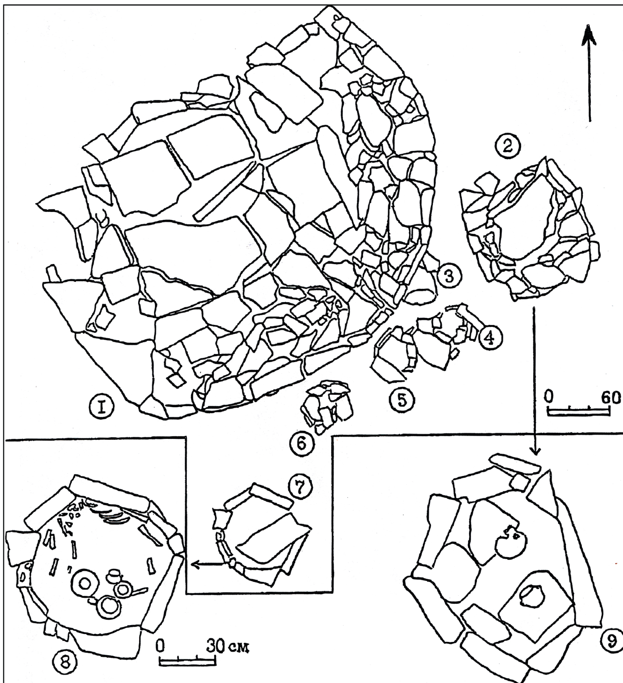
Рис 16. Могильник Гинчи. Планы склепа №9 (1), детских гробниц №№ 1–2 (2, 9 и 7, 8) и кувшинных погребений №№ 11–14 (3–6). По М.Г. Гаджиеву
