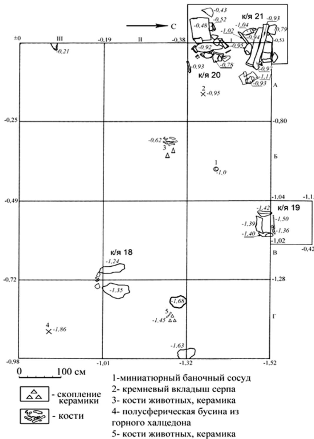
Рис. 11. Акярский могильник. Раскоп 2004 г. Общий план (слой 2)
