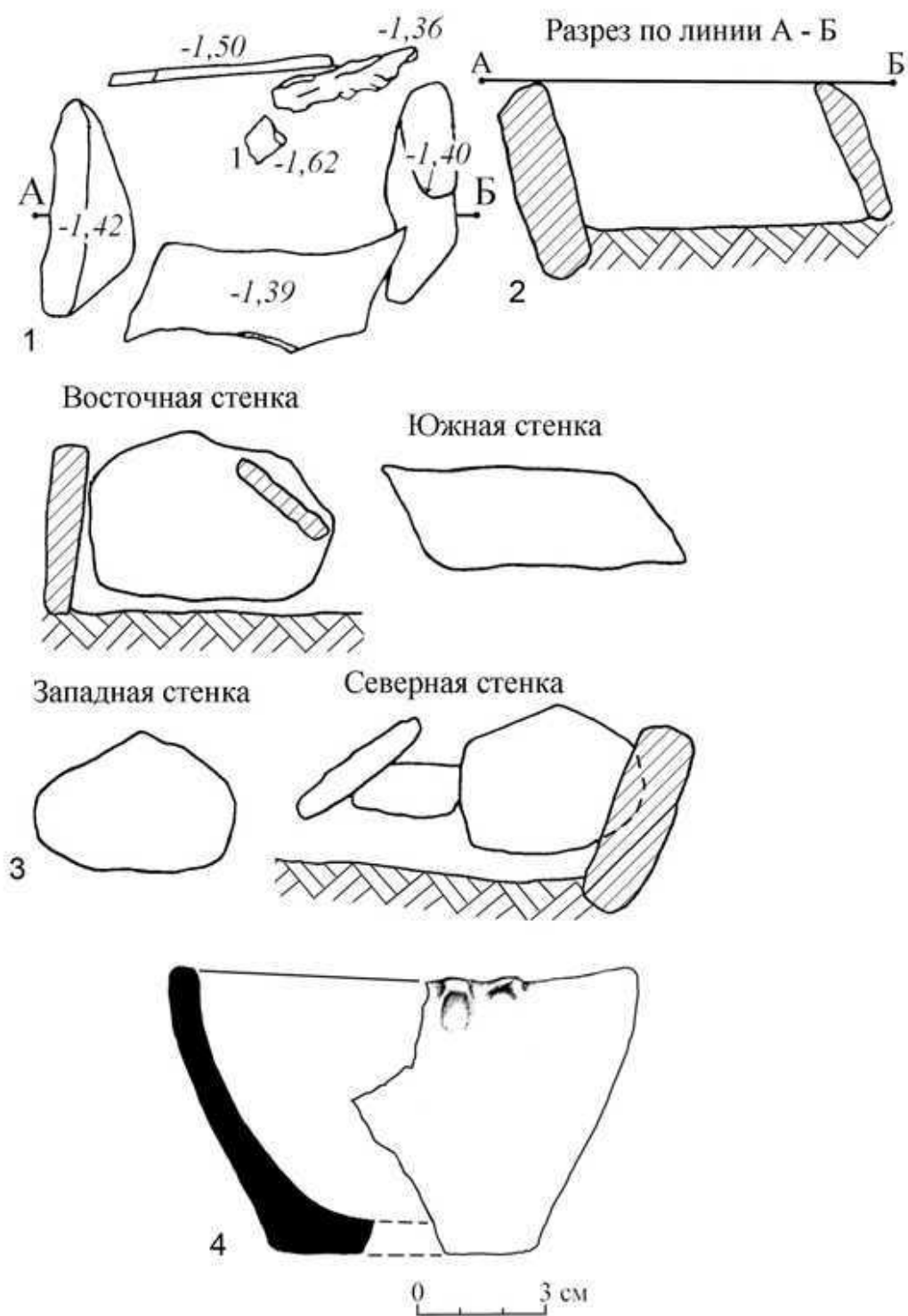
Рис. 15. Акярский могильник. Каменный ящик № 19 (№ 2, 2004 г.). 1 – план; 2 – разрез по линии А – Б. 3 – фасы стенок каменного ящика. 4 – миска.
